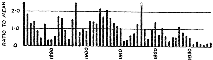
उत्तर डेकोटा, ग्रांड फोर्क्स पर रेड नदी। (औसत, १.२१ इंच। समय १८८२-१९३६)
